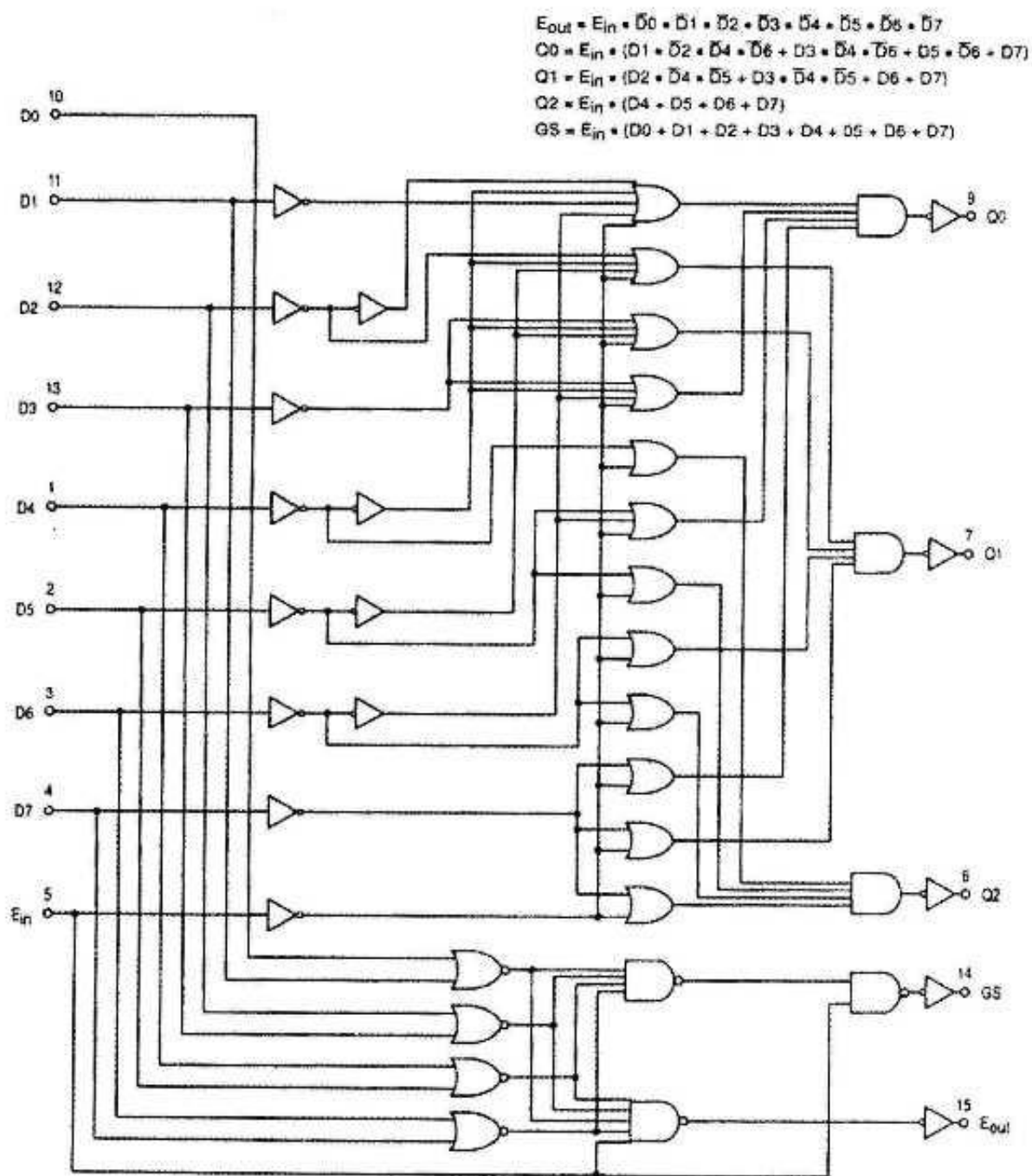
Функциональная схема
